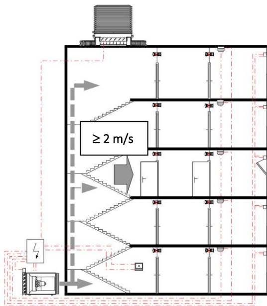
Kriterium Geschwindigkeit
