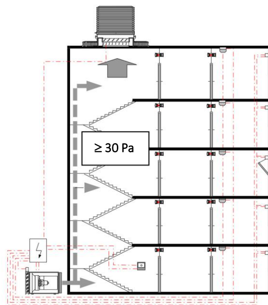
Kriterium Druck
